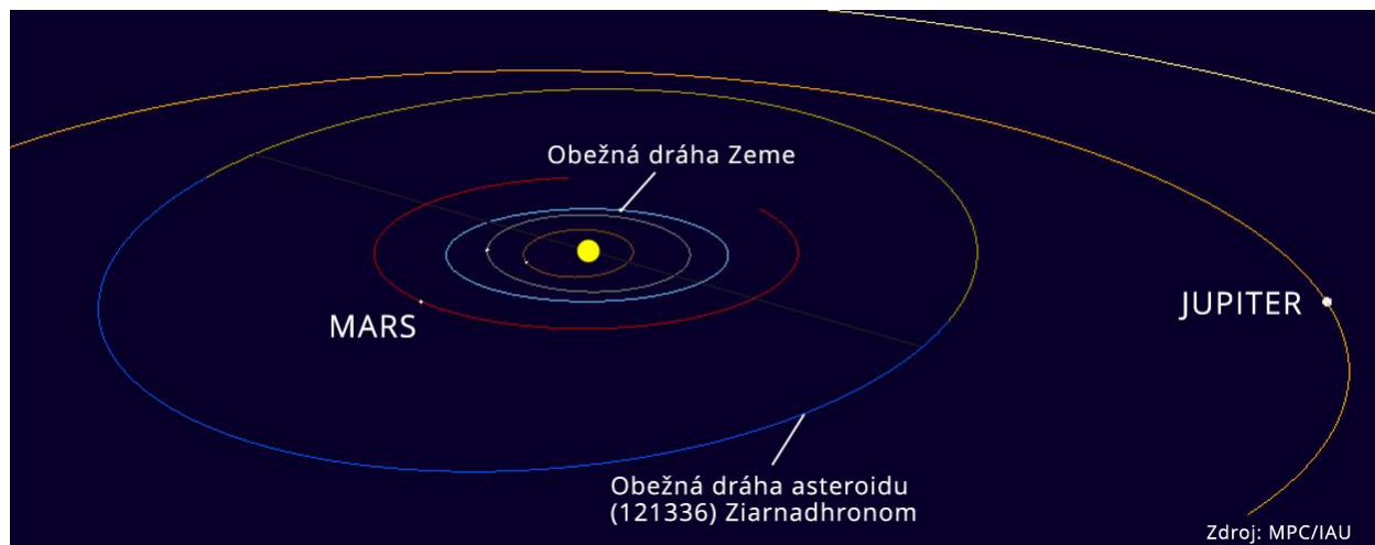
Schematické zobrazenie polohy obežnej dráhy asteroidu (121336) Ziarnadhronom v slnečnej sústave
